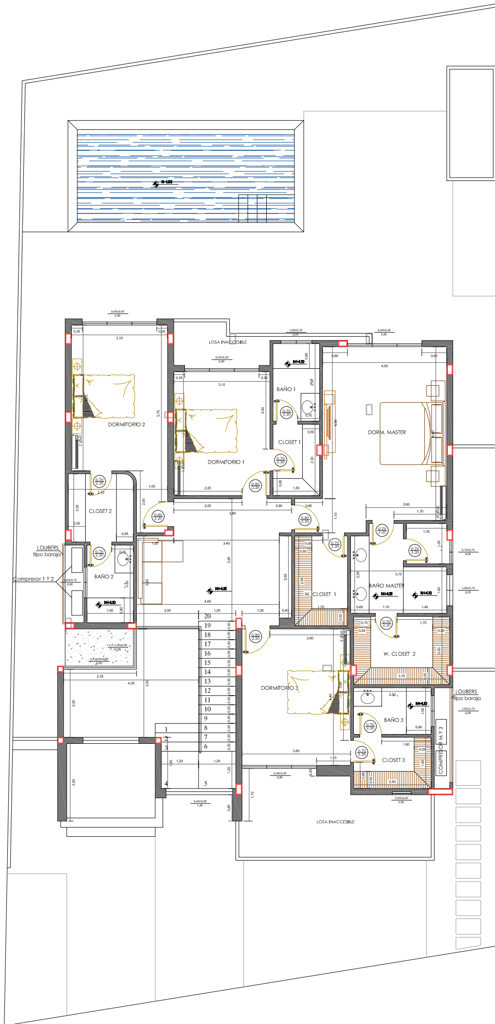
PLANTA ALTA
